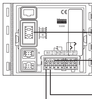
Module clavier 353000
